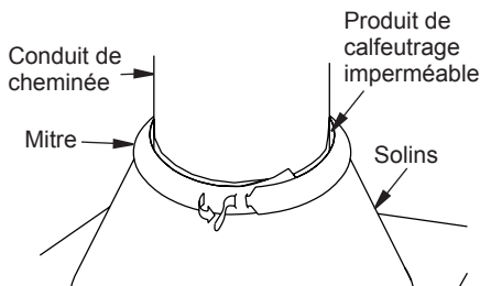
Figure 16 - Mitre
