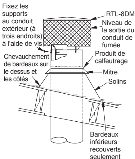
Figure 17 - Terminaison
