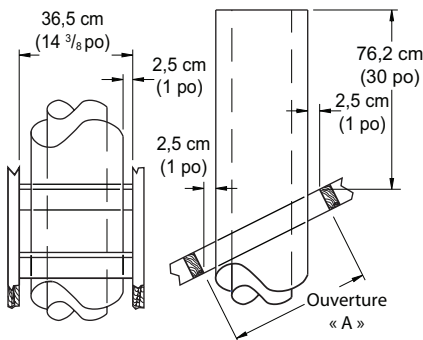
Dimensions Minimales
