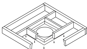
Figure 13 - Entretoise de pare-feu dans le cas d'un espace habitable au-dessus d'un plafond
