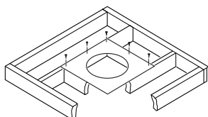
Figure 14 - Entretoise de pare-feu dans le cas d'un grenier au-dessus d'un plafond
