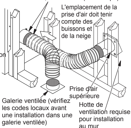
Figure 8 - Prêt-à-monter de gainé d'air extérieur
